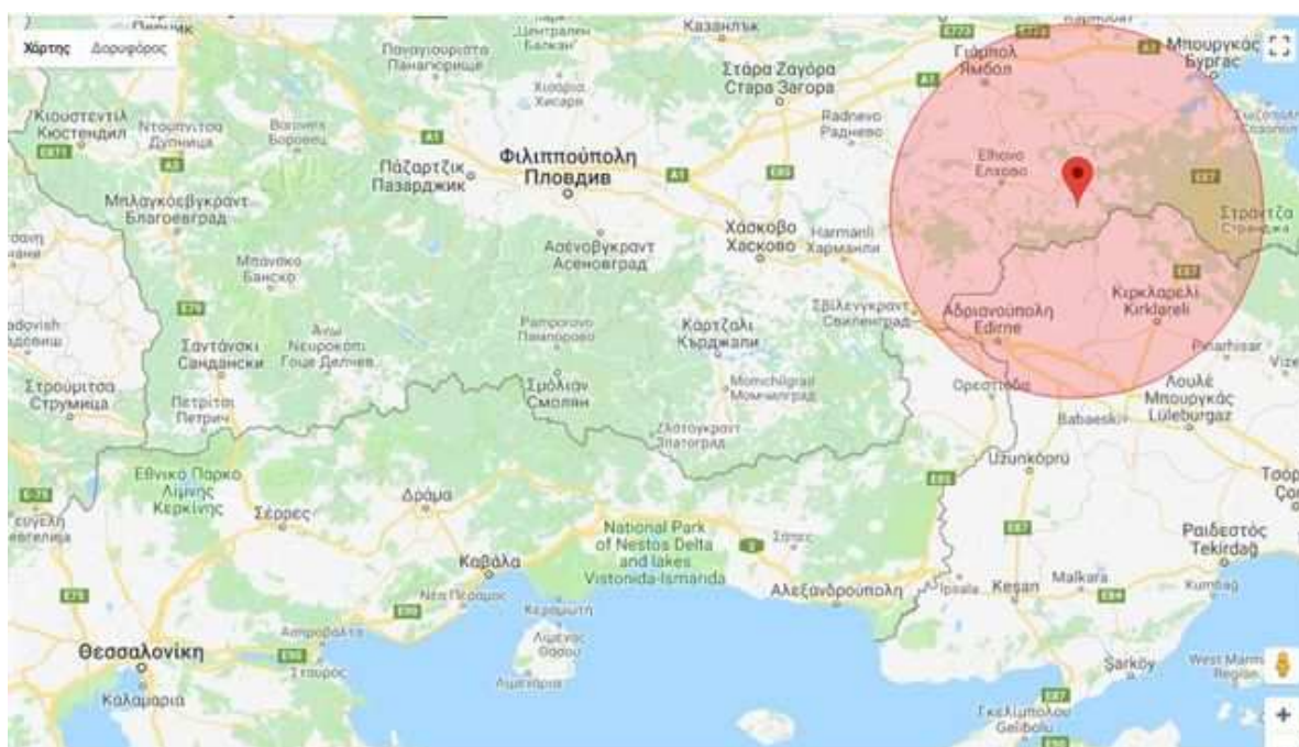
Εικόνα 2. Εστία Πανώλους Μικρών Μηρυκαστικών στη Βουλγαρία με ακτίνα 65 χλμ.
