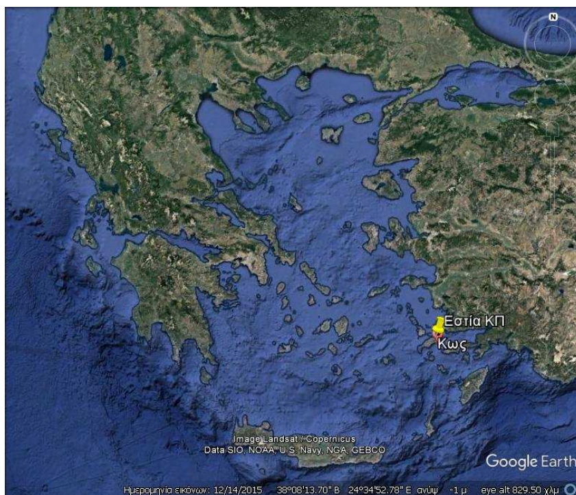
Εικόνα 1. Εστία ορομετατροπής ΚΠ στη Νήσο Κω.
