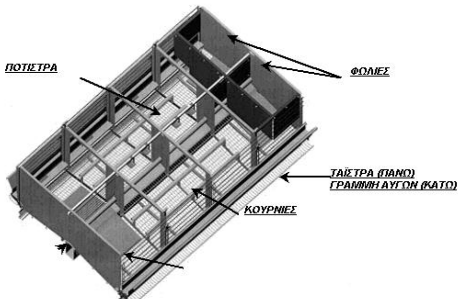
ΣΧΗΜΑ ΔΥΟ (2) ΕΜΠΛΟΥΤΙΣΜΕΝΩΝ ΚΛΩΒΩΝ
