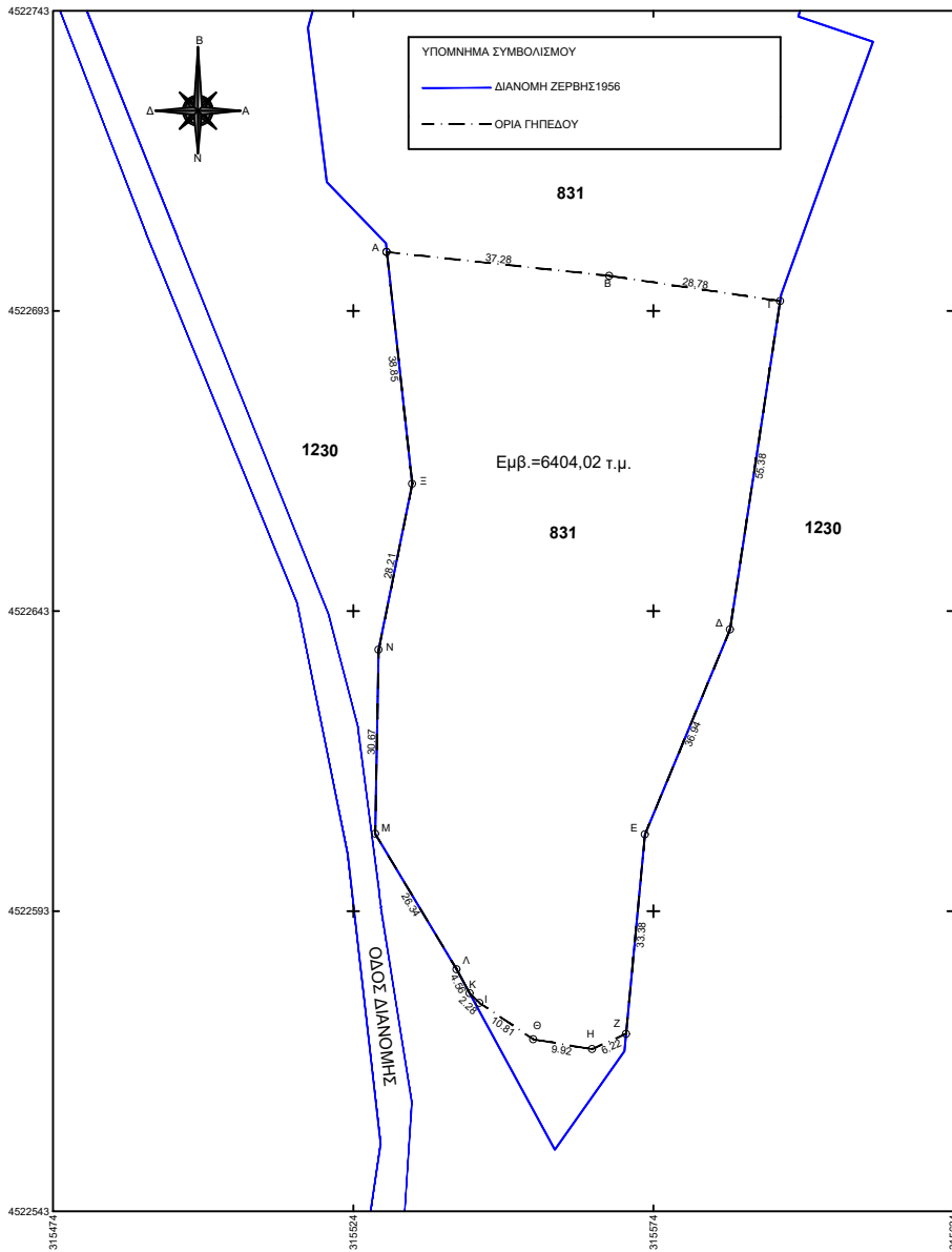
Πίνακας Συντεταγμένων ΕΓΣΑ των κορυφών του Α,Β,Γ.....Ξ Εμβαδόν τετραγώνου = 6404.02 τ.μ. - Περίμετρος = 349.62 μ.
